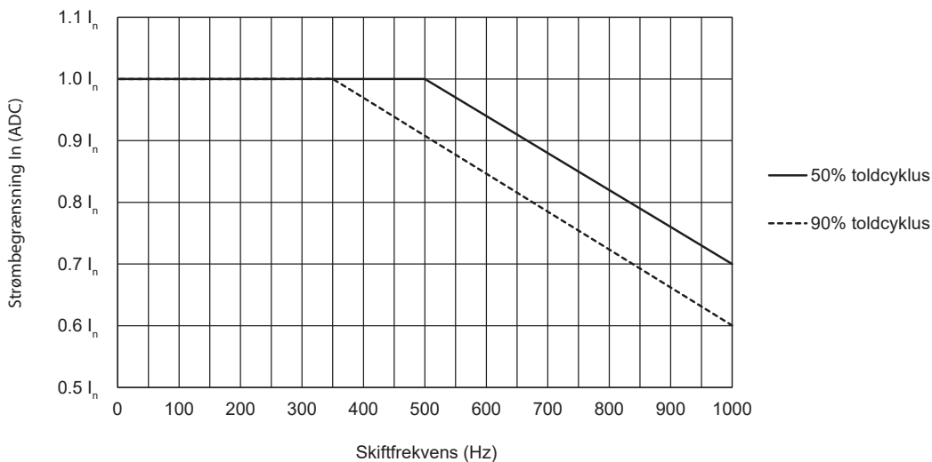
Fig. 4 Strømbegrænsning vs. skiffrekvens
